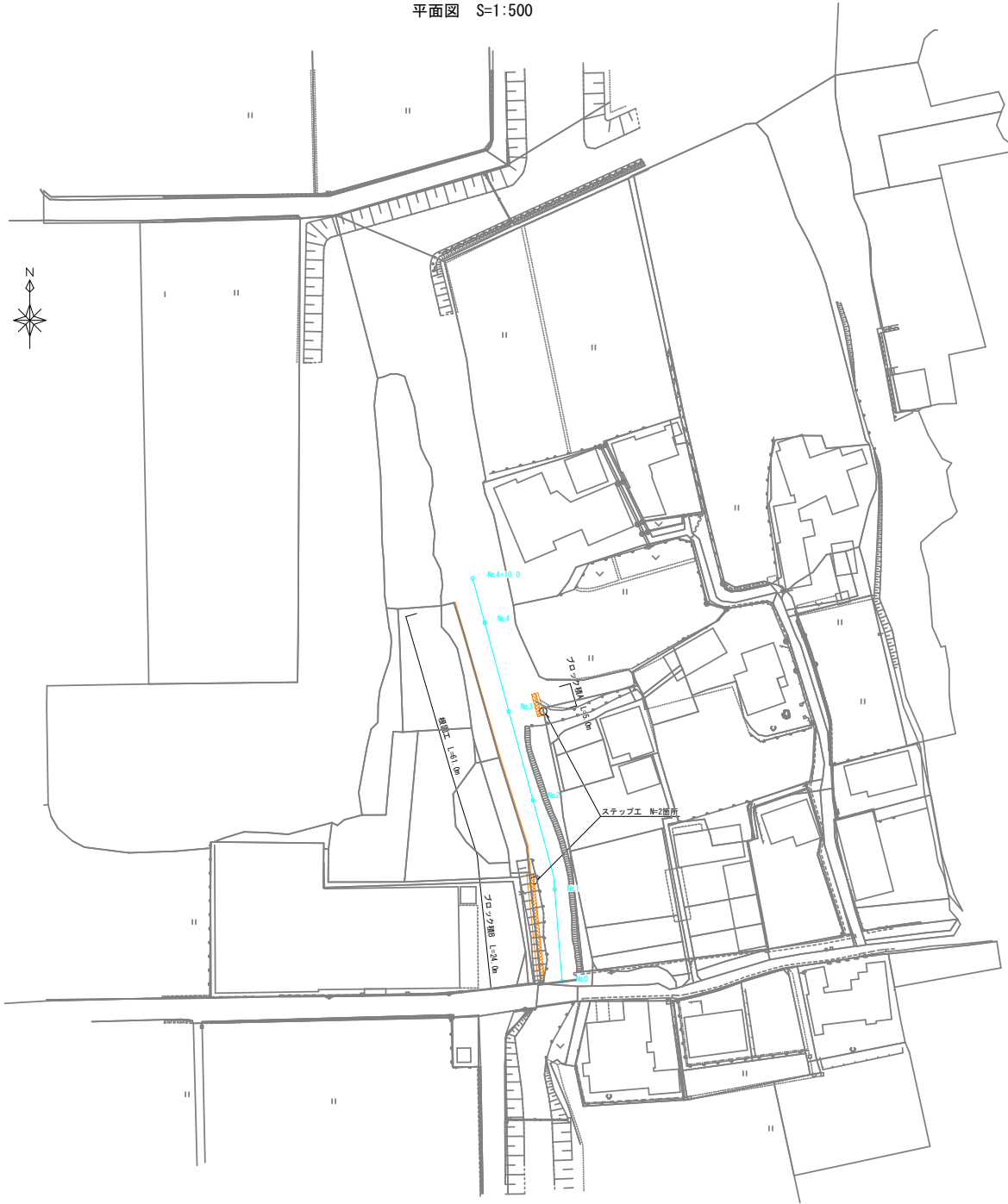
平面図 S=1:500
