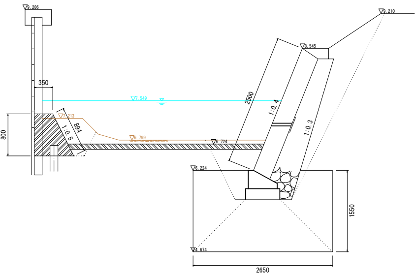
標準断面図 S=1:25 No.3付近
