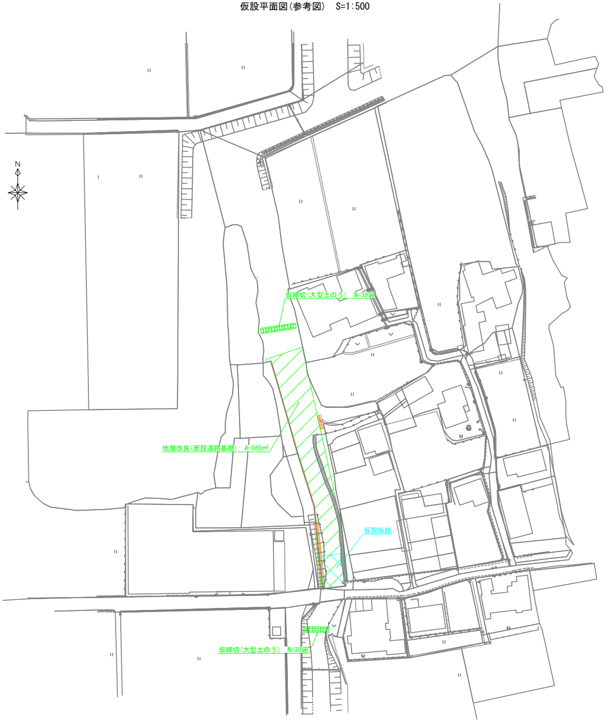
仮設平面図(参考図) S=1:500
