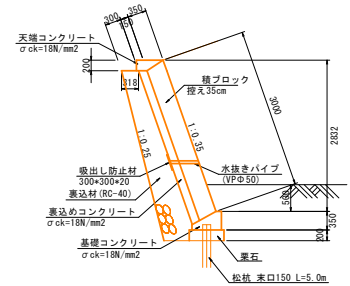
ブロック積工 S=1:50
