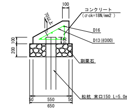
ブロック積基礎 S=1:20
