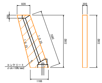
小口止工 S=1:50
