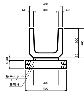
U形側溝断面図 S=1:10 300B
